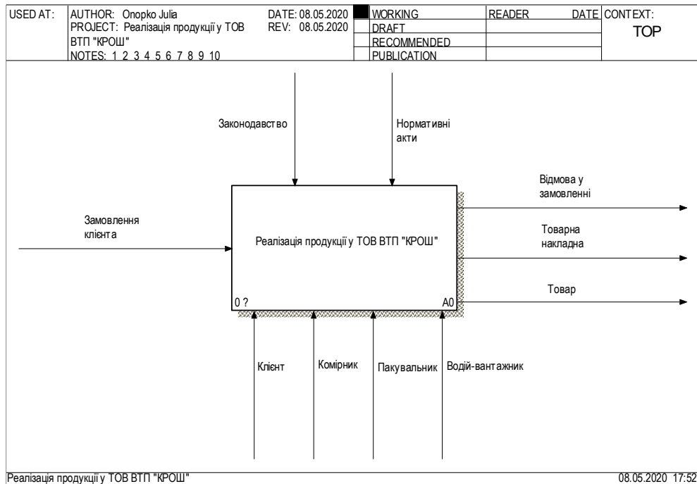
Рисунок 1.3 – Контекстна діаграма процесу реалізації продукції
